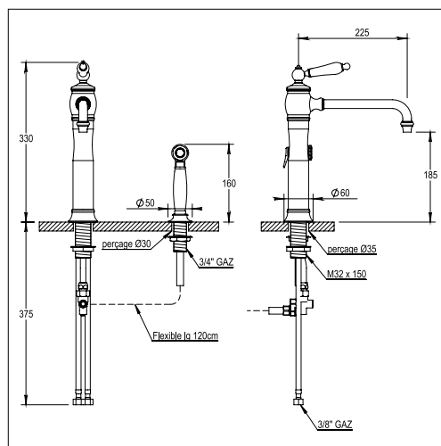
Mitigeur cuisine Eloïse avec douchette 02.723 Single lever sink mixer with handspray 02.723
