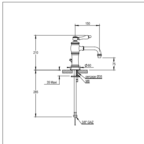
Mitigeur lavabo Eloïse 02.708 Single lever basin mixer 02.708
